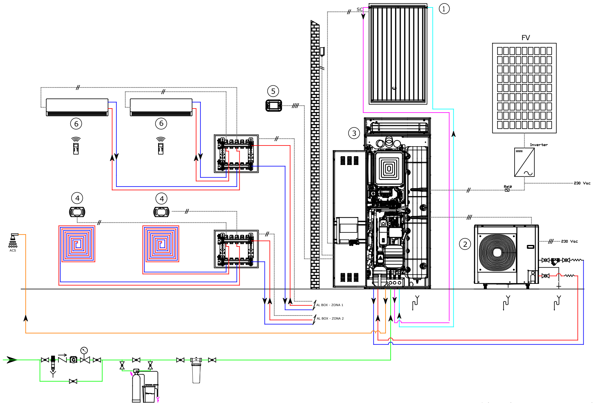
Schema di impianto puramente indicativo
